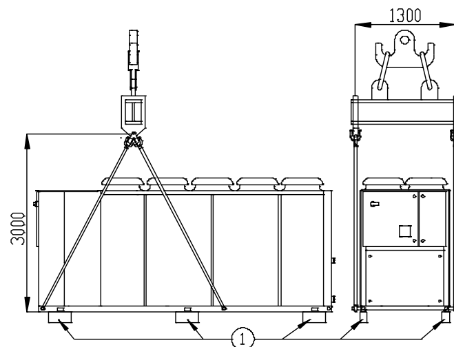
Unité à 4 points de levage
