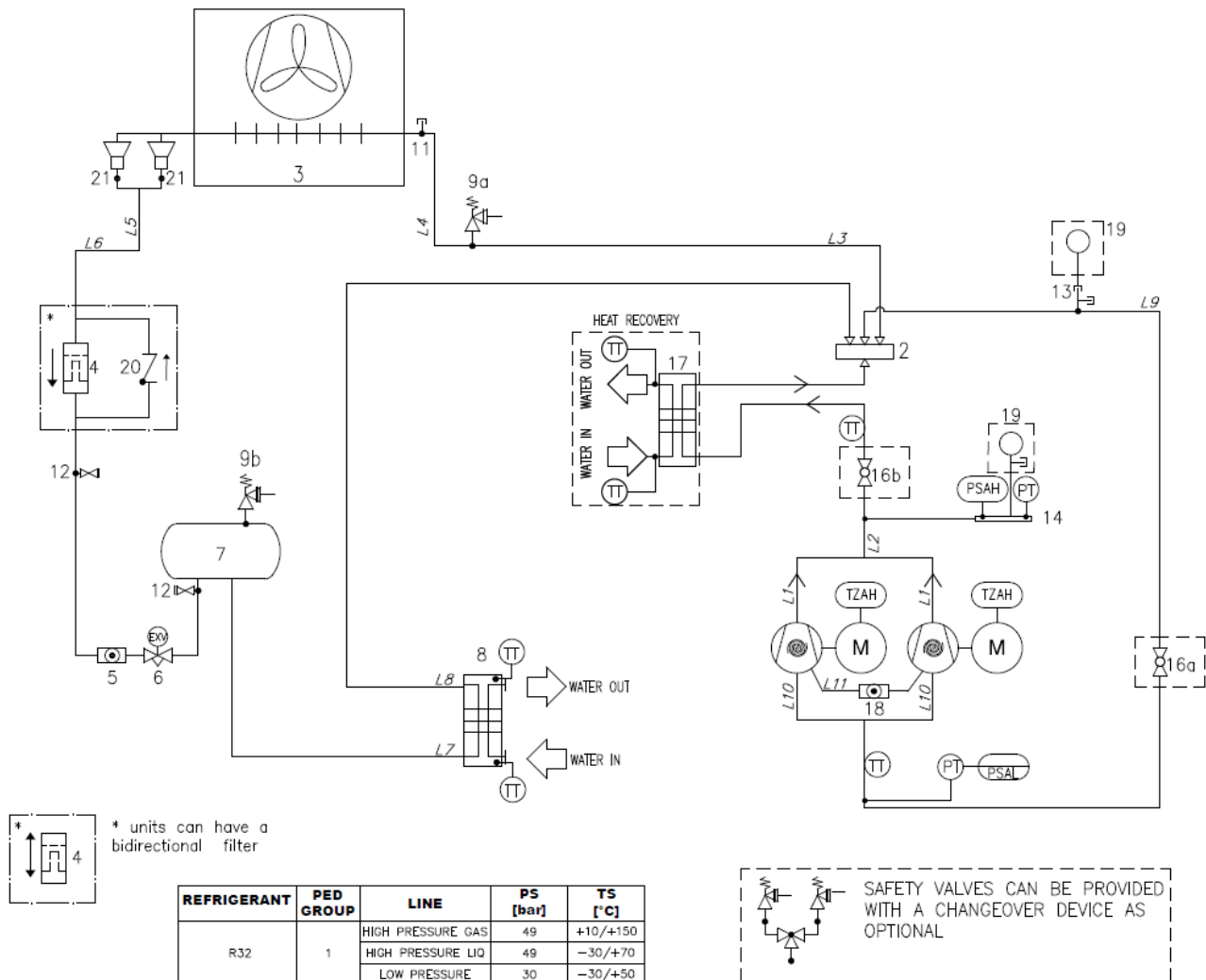
Fig. 19 - Schéma de tuyauterie de réfrigérant EWYTxx5B d'une unité à circuit unique (P&ID)
