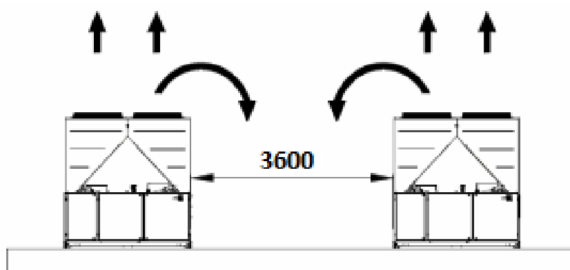
Fig. 3 - Encombrement minimal
