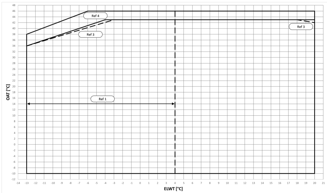
Fig. 12 - Limites opérationnelles du mode refroidissement EWYTxx5B-X
