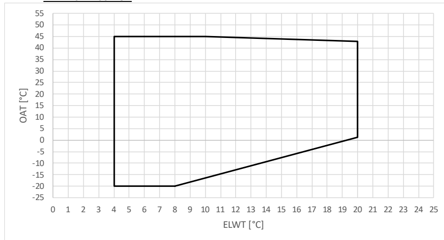
PLAGE DE FONCTIONNEMENT EN REFROIDISSEMENT - EWYT_CZ EWYT021-064-CZ
