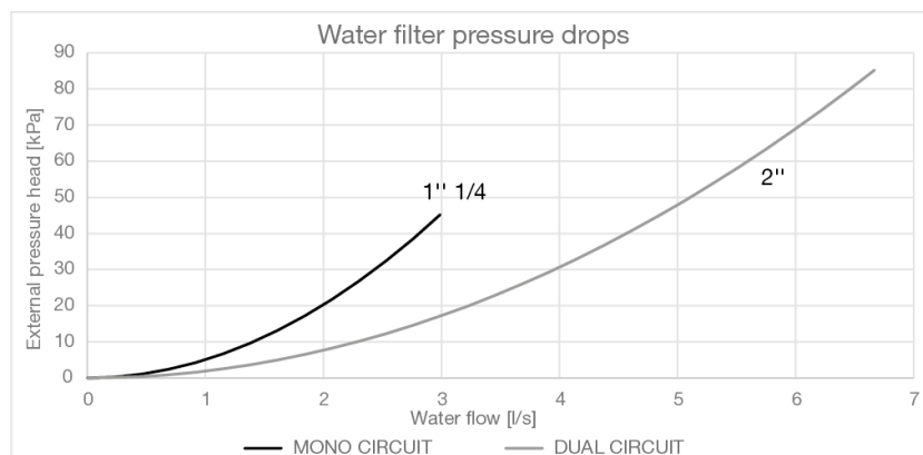
Figure 15 – Pertes de charge du filtre à eau
