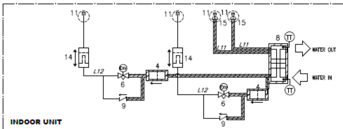
Figure 27 – Schéma du circuit de réfrigérant (P&ID) pour circuit DOUBLE unité intérieure EWYT-CZ
