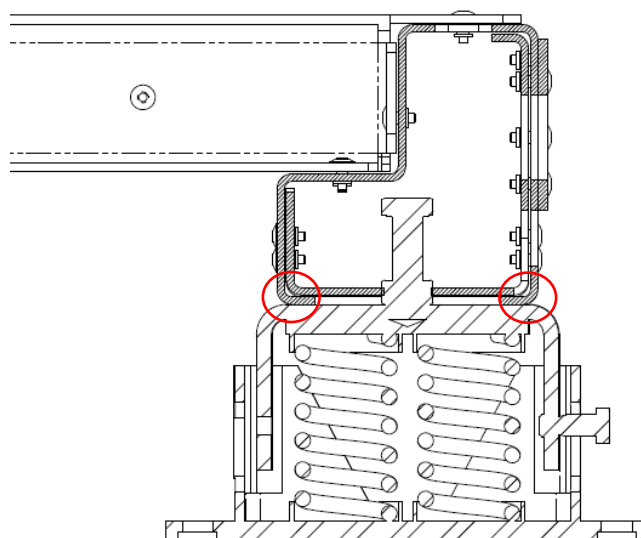
Fig. 12 Montage d'éléments anti-vibrations (fournis en option)
