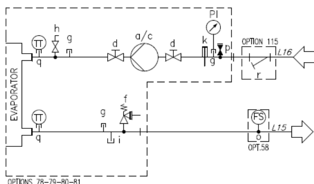
Fig. 13 – Diagramme hydraulique (opt. 78-79-80-81/134-135-136-137)
