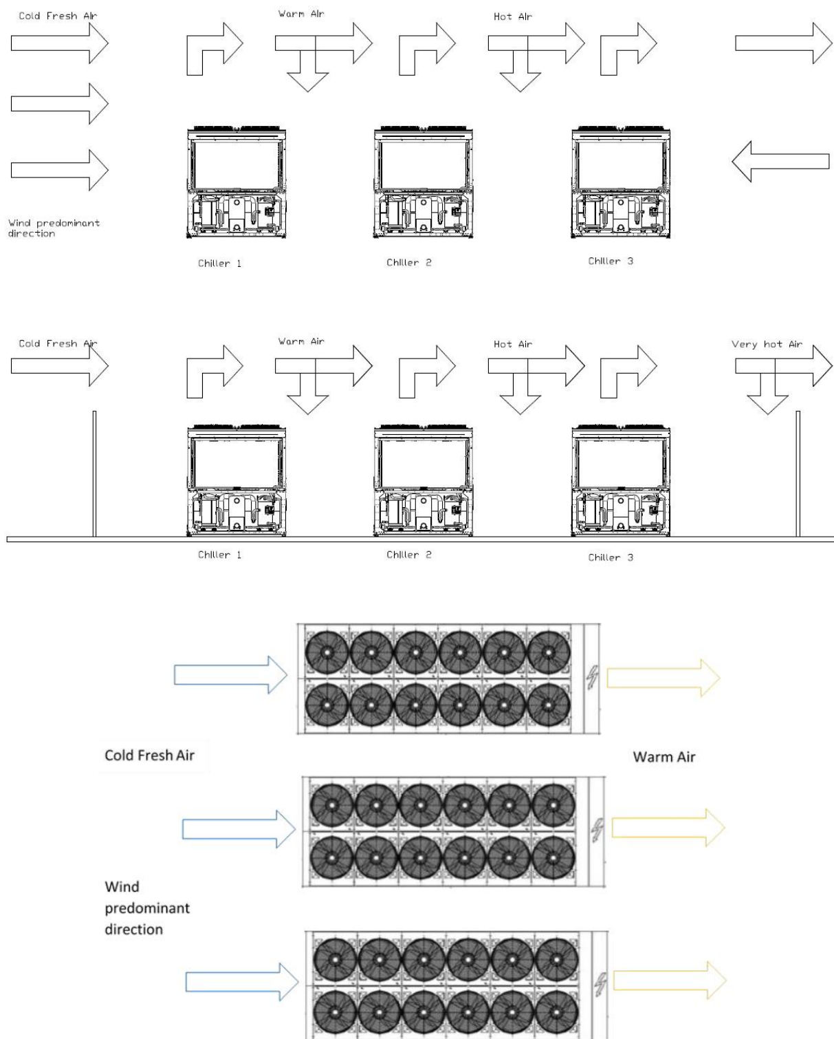
Fig. 11 – Installation de refroidisseurs multiples
