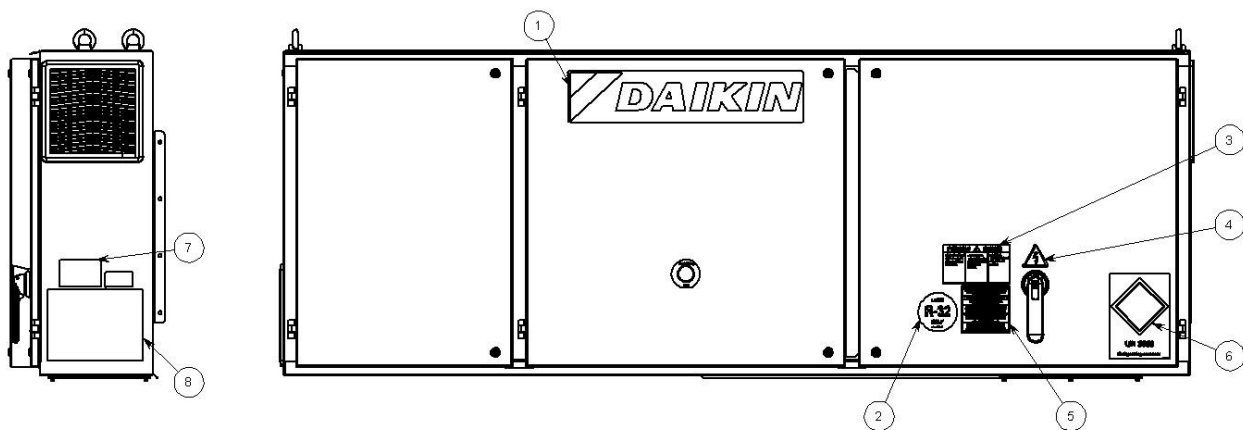
Fig. 15 – Description des étiquettes appliquées sur le Table électrique
