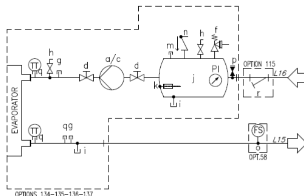
Fig. 13 – Diagramme hydraulique (opt. 78-79-80-81/134-135-136-137)
