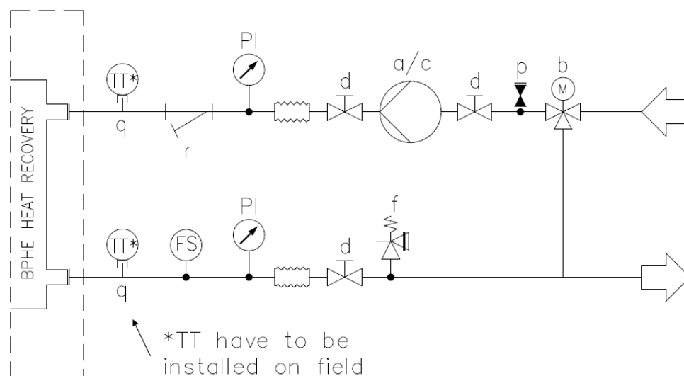
Fig. 14- Raccordement de la tuyauterie d'eau pour les échangeurs de récupération de chaleur (pression maximale de 20 bar)
