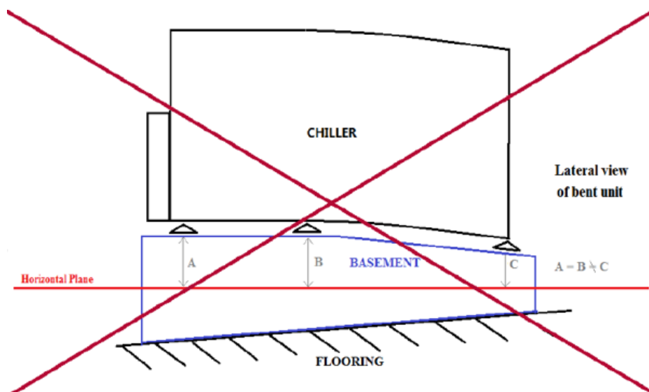
Fig. 9 – Nivellement de l'unité
