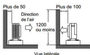
Vue latérale
