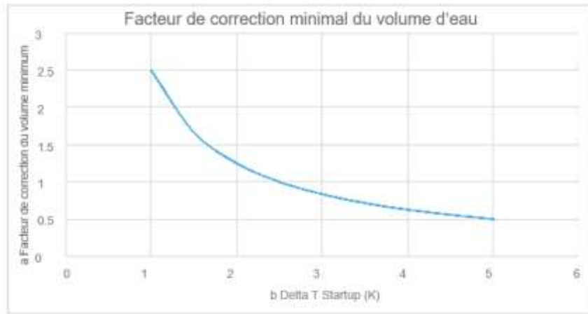
Illustration 17 - Facteur de correction du volume d'eau minimal
