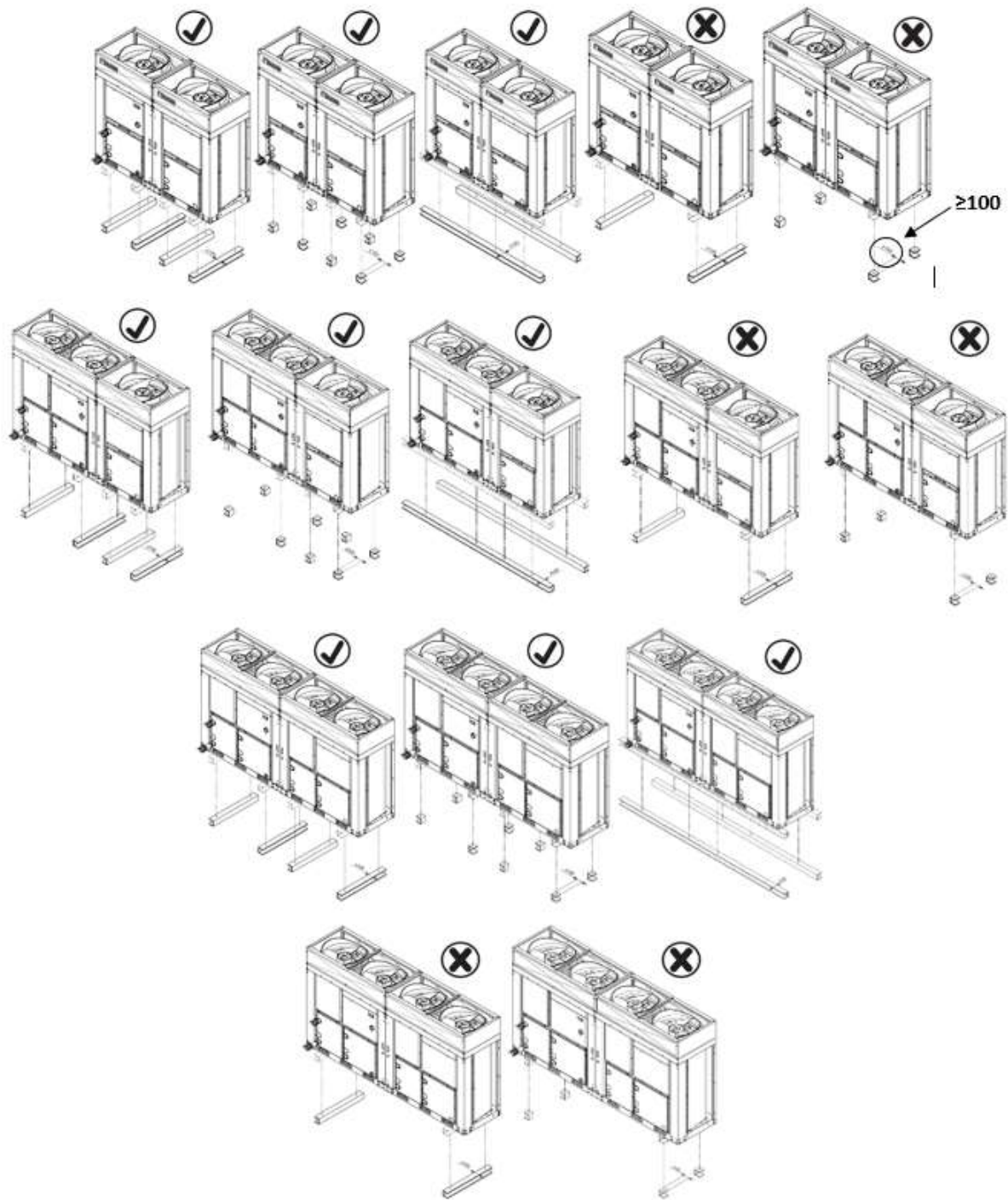
Illustration 4 – Mise en place de l'unité DUAL
