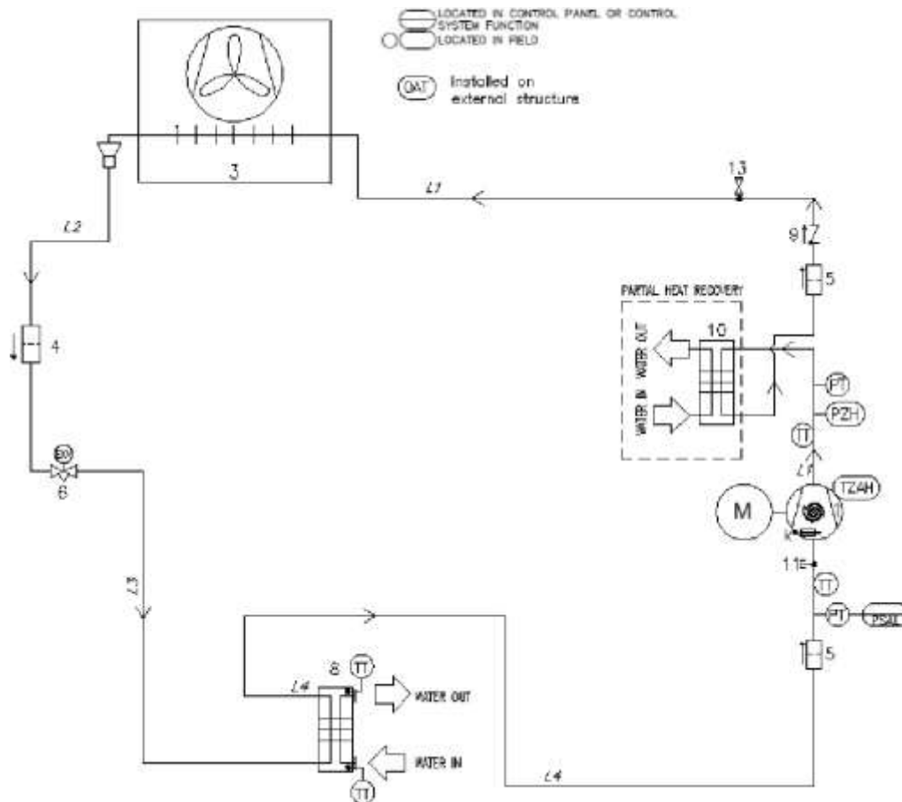
Illustration 20 - Schéma du circuit de réfrigérant (P&ID) pour circuit MONO unité EWAT-CZ
