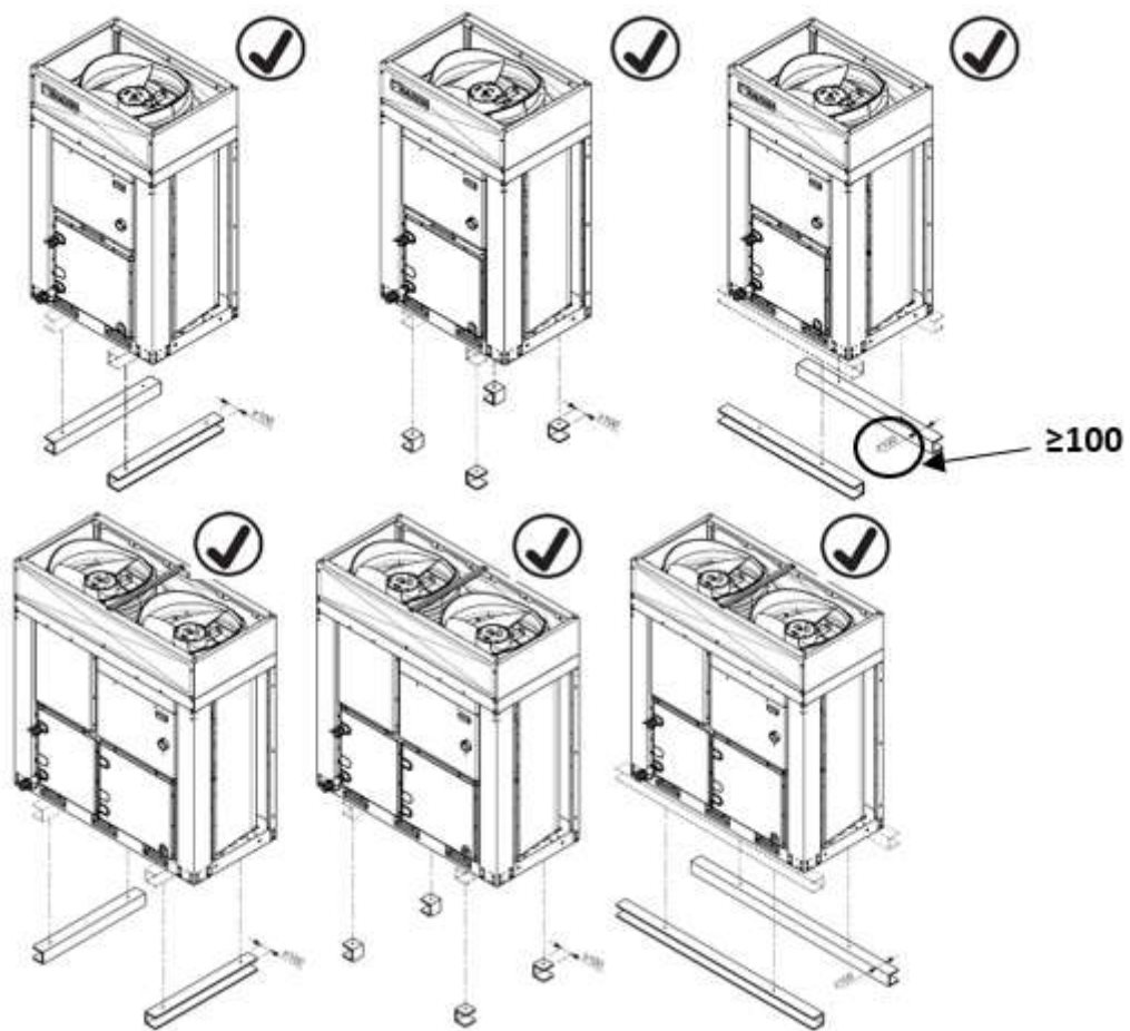
Illustration 3 – Mise en place de l'unité MONO
