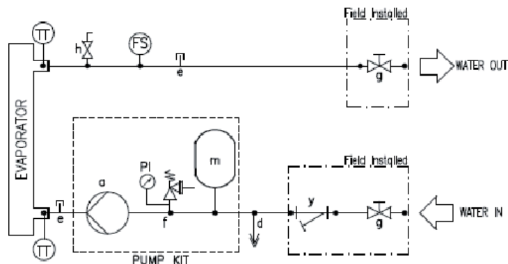
Illustration 10 – Schéma hydraulique
