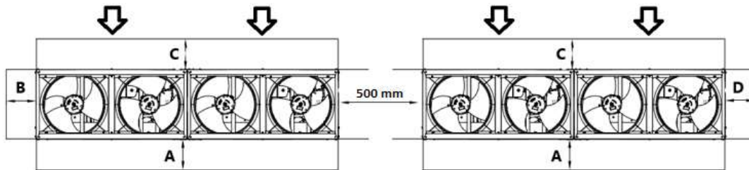
Illustration 7 –Unités installées côte à côte le long de leurs côtés les plus courts, B ou D
